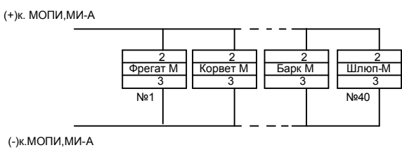
Схема адресного шлейфа
