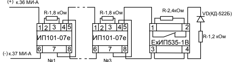
Схема шл. пт.
