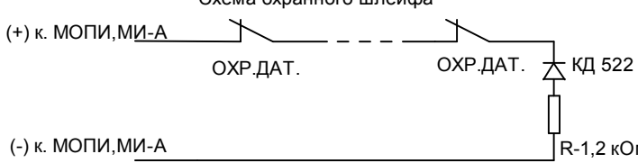
Схема охранного шлейфа
