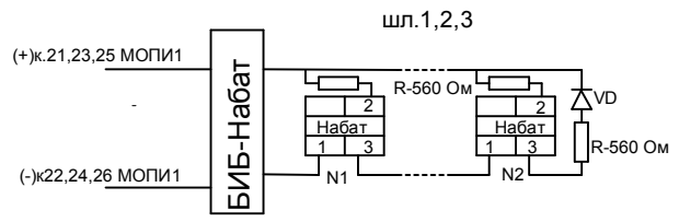
шл. ПТ. 1.2 (Напр. 1-Маш. зал)
