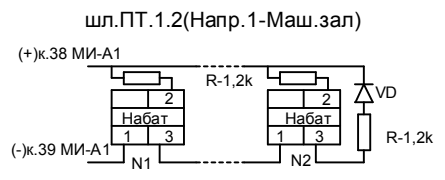
Схема шлейфов
