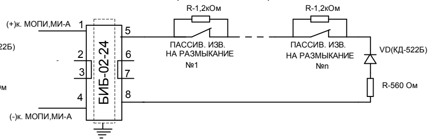
Схема шл. пт.
