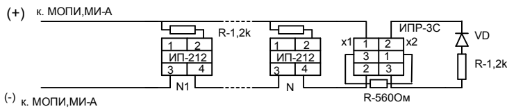
Схема шлейфов МОПИ и МИ-А
