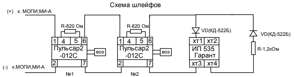
Схема адресного искробезопасного шлейфа
