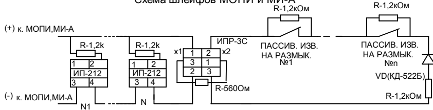
Схема шлейфов МОПИ и МИ-А
