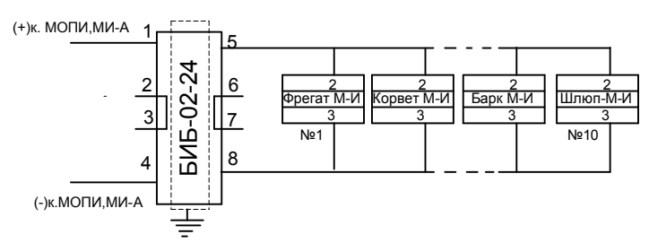
Схема шлейфа пассивного искробезопасного
