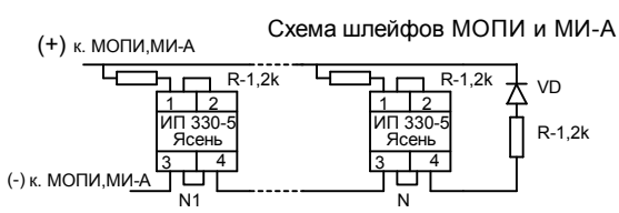
Схема шл. 1
