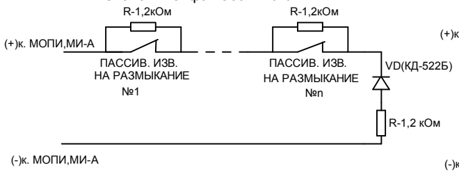
Схема шлейфа пассивного
